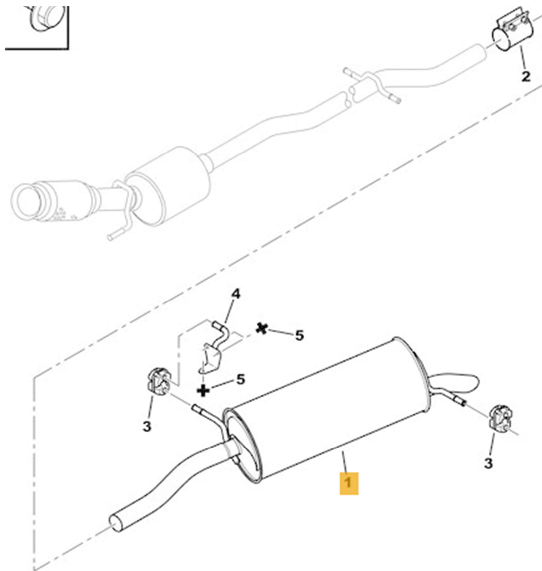
Original 55mm udstødning. DPF monteres efter katalysator vha. clamps/muffe.
